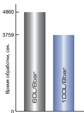
Рис. 1: 20% сокращение времени за счет оптимизированной подачи охлаждения
