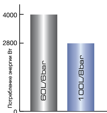
Рис. 2: 30% сокращение потребления энергии за счет оптимизированной подачи охлаждающего средства
