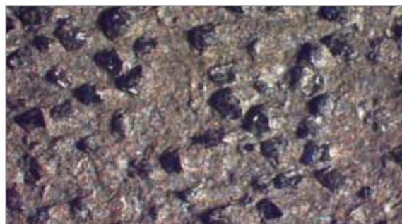
Рис. 2: заточенный абразивный слой
